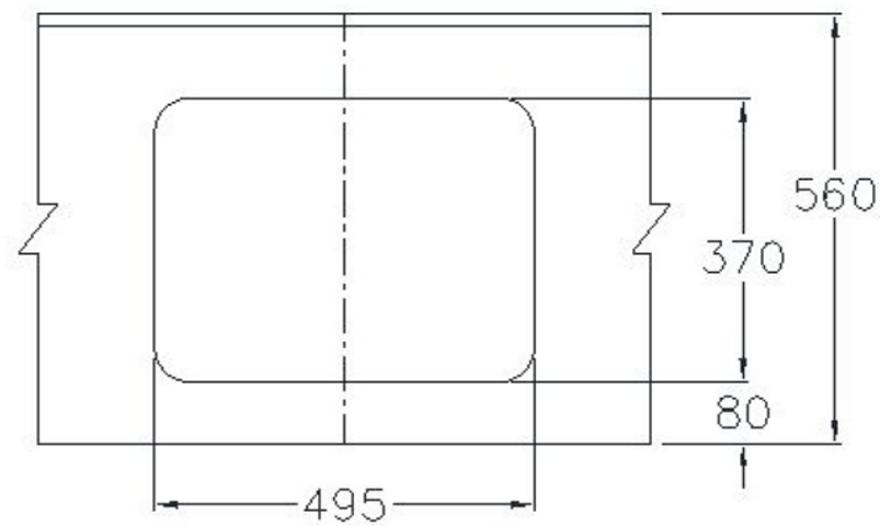
枱面挖孔尺寸圖
