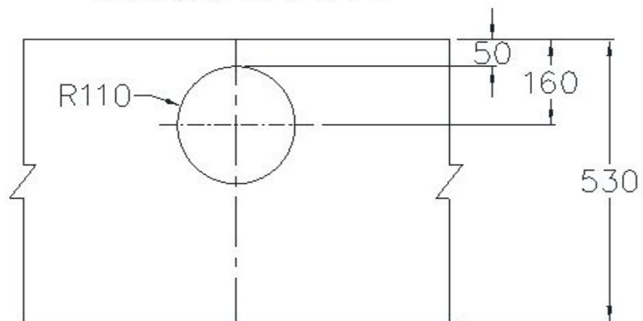
枱面挖孔尺寸圖
