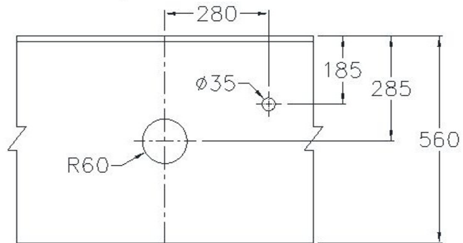
枱面挖孔尺寸圖
