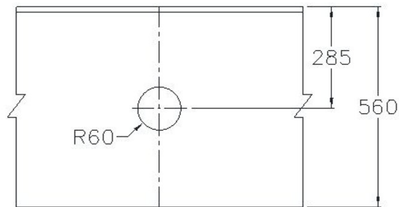
枱面挖孔尺寸圖
