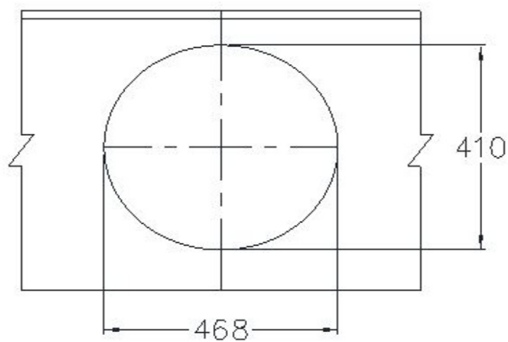
枱面挖孔尺寸圖
