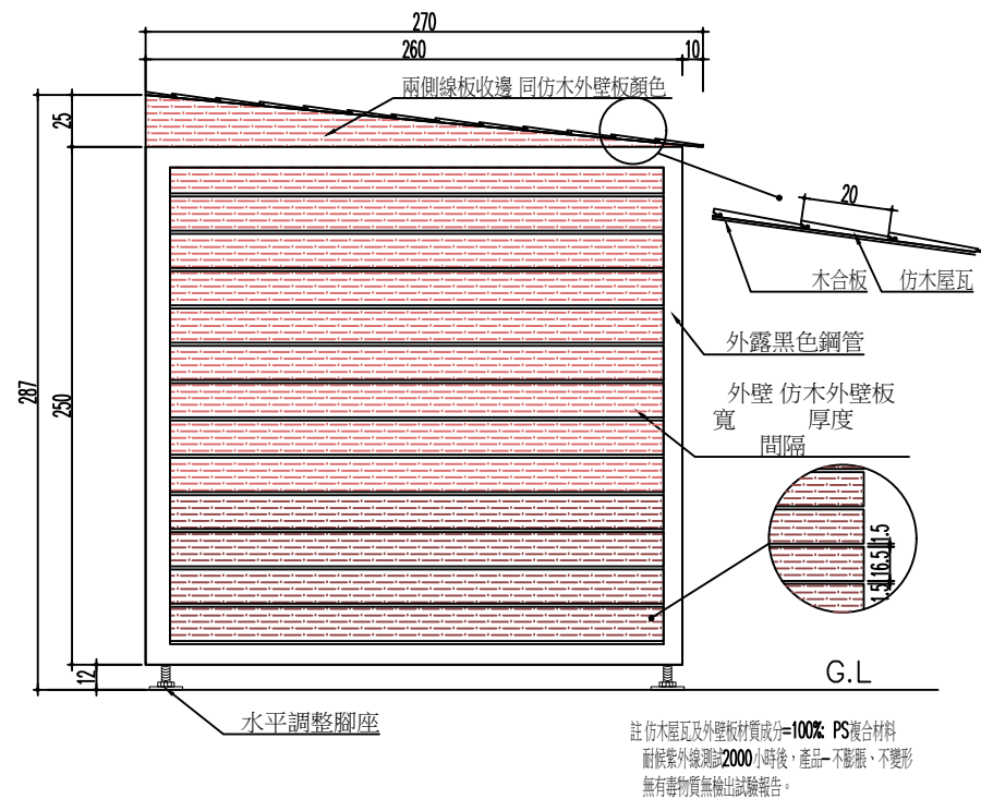
1 (無障礙) 左側立面圖 SCALE: 1/40
