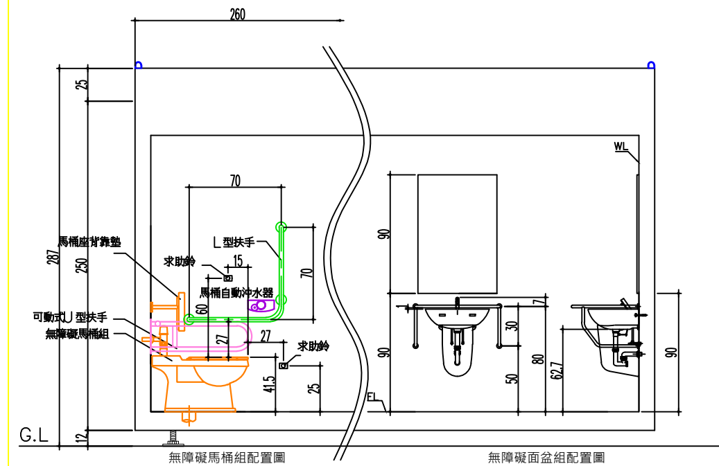
6 (無障礙) 立剖面圖 SCALE: 1/40
