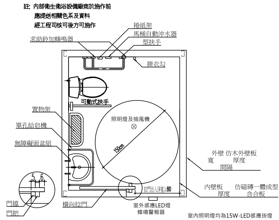
2 無障礙廁所平面配置圖 SCALE: 1/40
