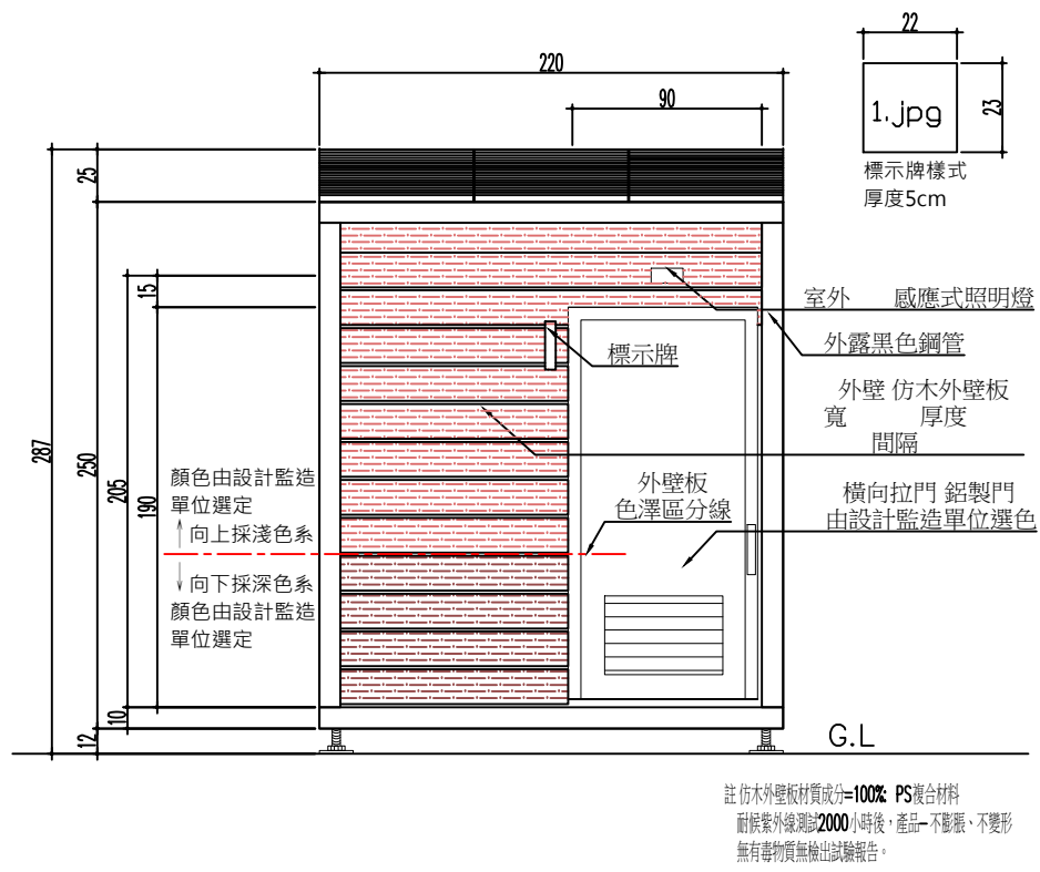
5 (無障礙) 正立面圖 SCALE: 1/40
