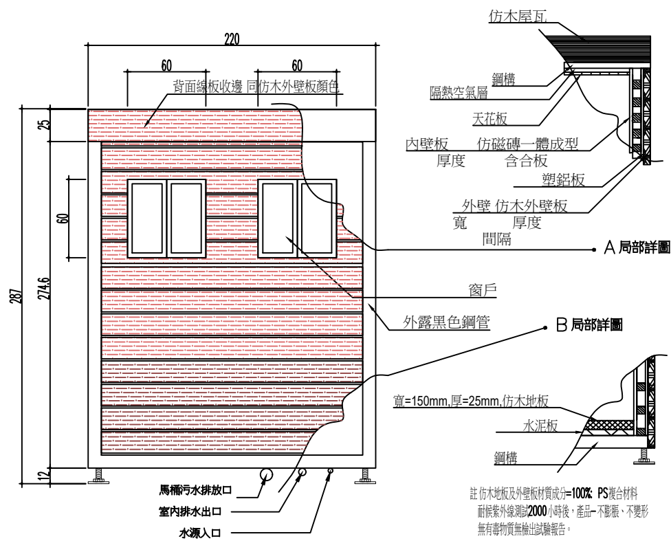
4 (無障礙) 背立面圖 SCALE: 1/40
